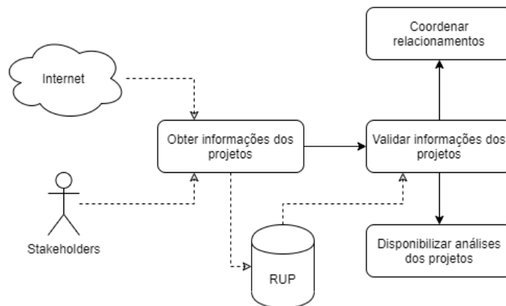
Figura 1. Fluxo operacional do OUP
