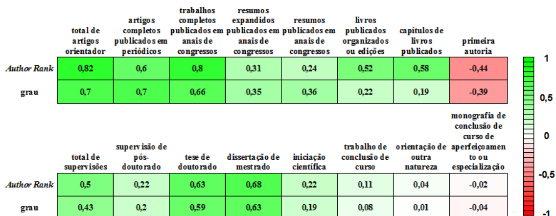
Figura 9. Correlação entre Author Rank e grau dos nós e as demais métricas
