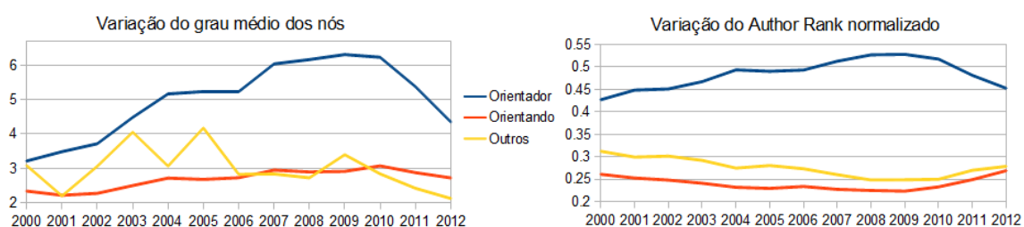
Figura 7. Variação do grau e do Author Rank de 2000 a 2012
