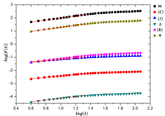
Fig. 5. Valores do logaritmo da função F_{DFA} em função do logaritmo do tempo, dado em semanas.
