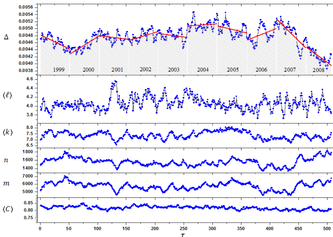
Fig. 2. Evolução dos índices das janelas temporais entre 1999 e 2008. As linhas retas no gráfico de \Delta representam o melhor ajuste linear para janelas de 1 ano
