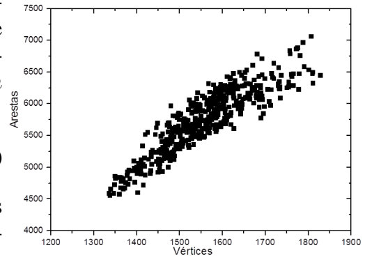
Fig. 4. O número de vértices cresce em média proporcionalmente ao número de arestas
