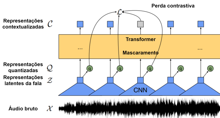
Figura 1. Arquitetura do Wav2vec 2.0 - Adaptado de [Baevski et al. 2020b].
