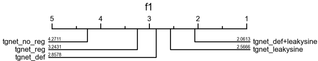
Figura 8. Diagrama de diferença crítica do estudo de ablação da influência de cada mecanismo agregado a arquitetura do TGNet.
