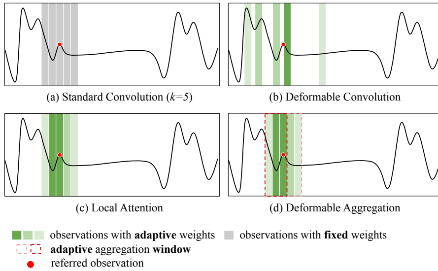
Figura 2. Comparação de diferentes mecanismos utilizados para extrair padrões temporais entre as observações de uma série temporal.
