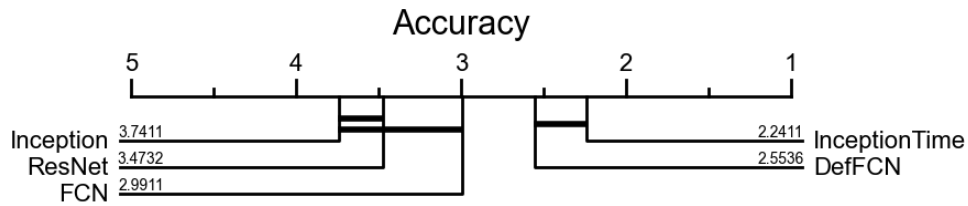
Figura 6. Diagrama de diferença crítica entre as redes para classificação de séries temporais e a DeformableFCN que utiliza convoluções deformáveis.
