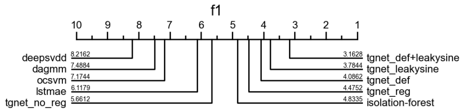
Figura 7. Diagrama de diferença crítica dos métodos de OCL. Os experimentos foram realizados nas variações de conjuntos de OCL a partir do repositório da UCR.
