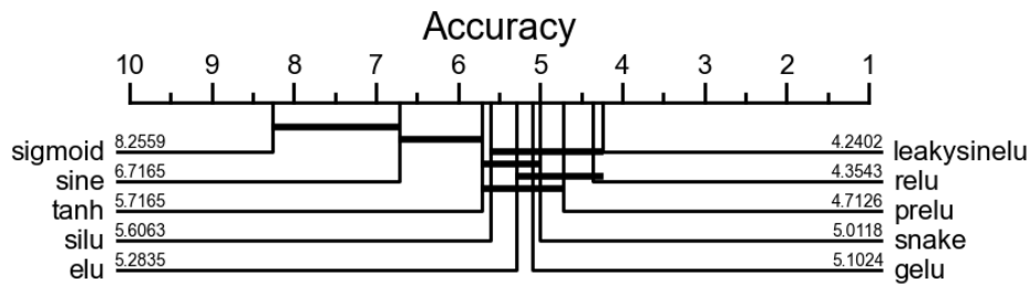
Figura 4. Diagrama de diferença crítica entre as ativações comparadas utilizando como base uma rede MLP [Wang et al. 2017].
