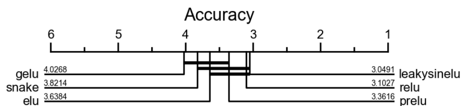
Figura 5. Diagrama de diferença crítica entre as ativações comparadas utilizando como base uma rede FCN [Wang et al. 2017].
