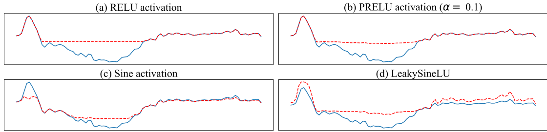
Figura 1. Comparação entre diferentes funções de ativação aplicadas a saída de uma camada de rede neural aplicada em uma série temporal.
