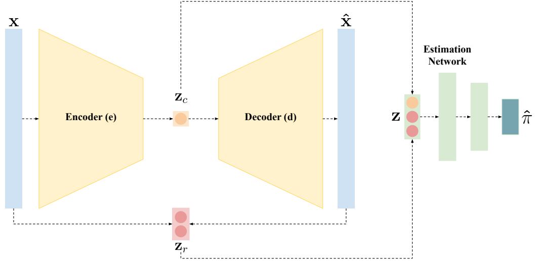
Figura 3. Visão geral da arquitetura do TGNet.
