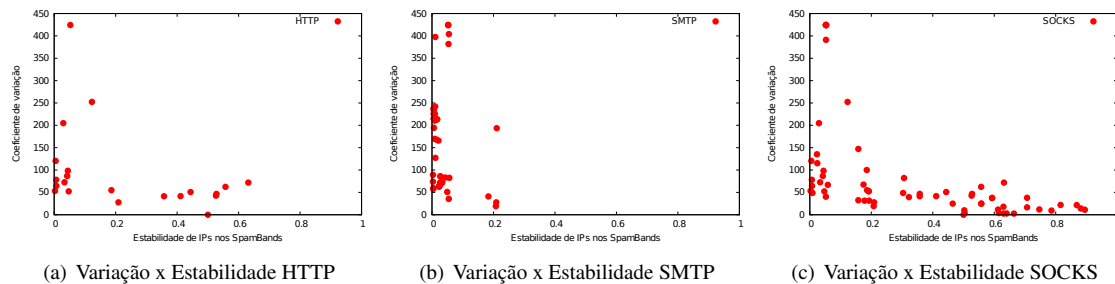
Figura 8. Estabilidade e desvio padrão relativo de IPs nos SpamBands , ao longo do dia, por protocolo
