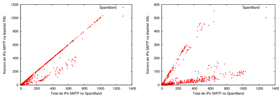
(a) Distribuição de IPs SMTP por IPs SMTP na PBL nos SpamBands (b) Distribuição de IPs SMTP por IPs SMTP na XBL nos SpamBands
