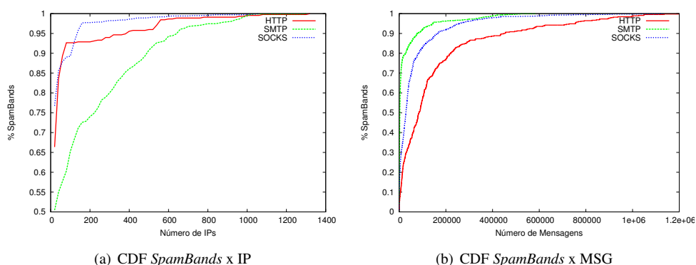
Figura 4. SpamBands em relação ao número de endereços IP e mensagens
