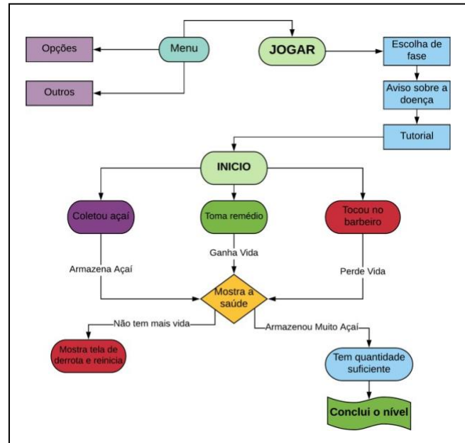
Figura 2. Fluxo do jogo.
