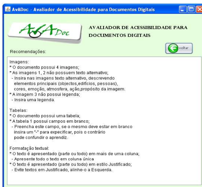
Figura 5. Relatório gerado pelo AvADoc
