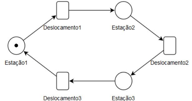
Figura 2: modelo GSPN de um sistema de transporte urbano via metrô.
