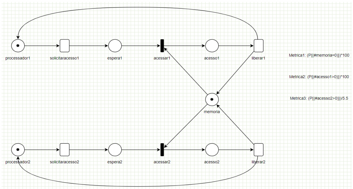
Figura 14: exemplo de exercício de modelagem de nível avançado.
