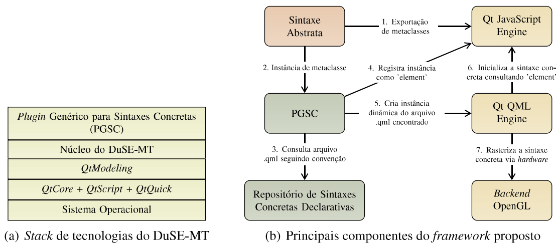
Figura 1. Stack de tecnologias (a) e principais componentes (b) utilizados no framework proposto.
