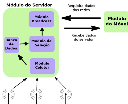
Figura 2. Arquitetura do Sistema
