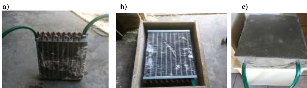
Figura 1. a) sistema de serpentinas para a circulação de água quente; b) serpentinas num molde de madeira para preenchimento com argamassa; c) molde preenchido com argamassa e mangueiras para conexão com as fontes de água quente e fria (Fonte: Rohr et al., 2017).
