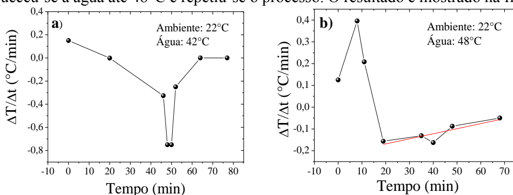
Figura 3. a) Taxa de variação da temperatura do piso térmico em função do tempo após desligar o aquecedor resistivo no momento em que a água da fonte quente atinge 42°C e b) após atingir 48°C.
