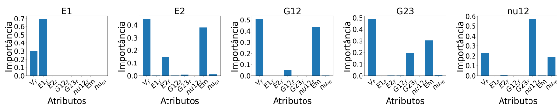
Figura 4. Importância das características do melhor modelo de árvores de decisão para cada uma das propriedades.
