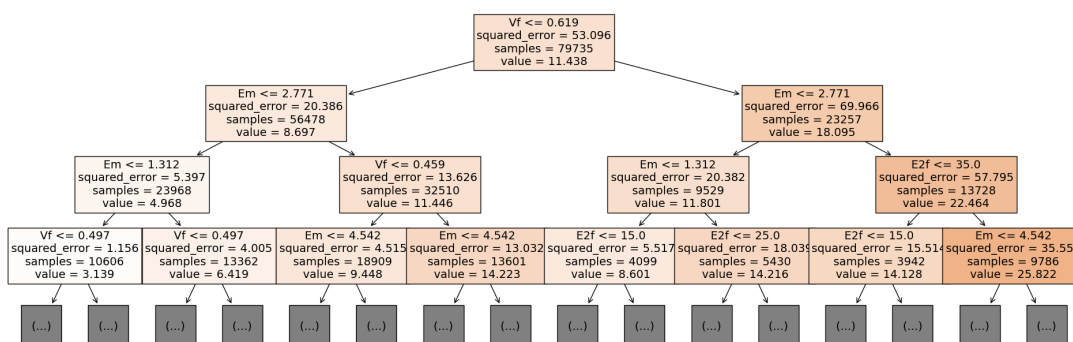
Figura 6. Visualização da árvore de decisão gerada para previsão da propriedade E2.
