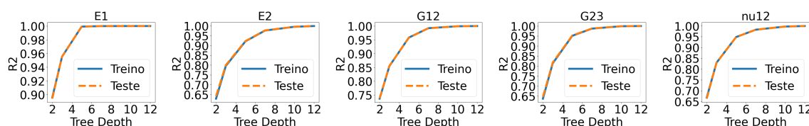
Figura 3. Complexidade Árvores de Decisão.
