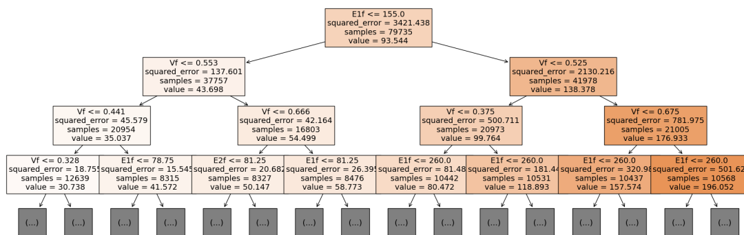
Figura 5. Visualização da árvore de decisão gerada para previsão da propriedade E1.
