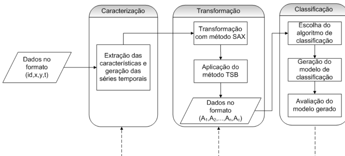
Figura 33: Visão geral do método TRACTS
