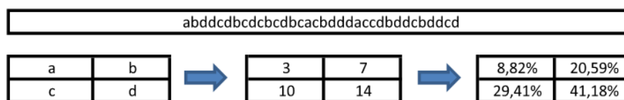
Figura 4: Geração de uma matriz TSB
