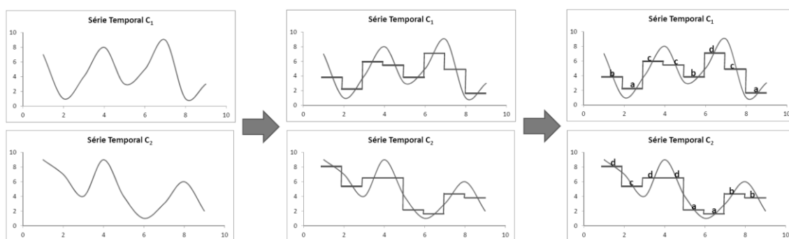
Figura 22: Aplicação do método SAX em duas séries temporais
