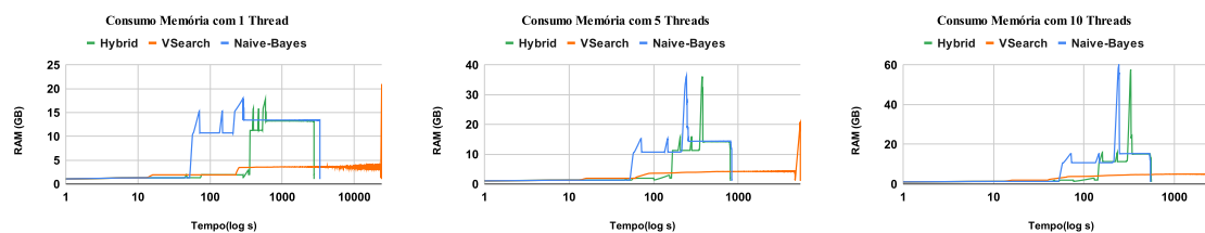
Figura 3. Comparação do consumo de memória entre os algoritmos.
