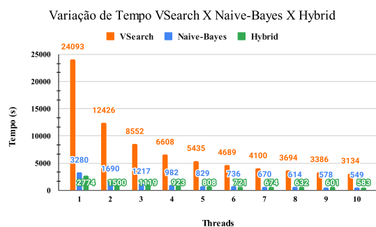
Figura 1. Tempos médios de execução.
