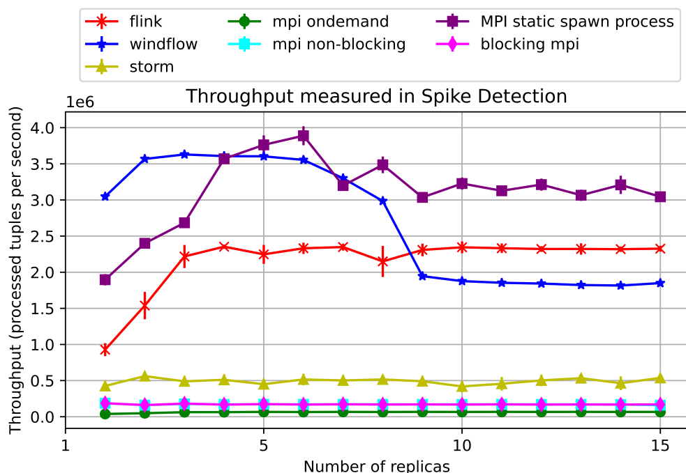
Figura 2. Throughput de SD em diferentes réplicas de Moving Average.
