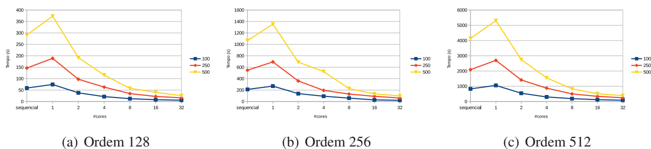
Figura 1. Tempo de execução (s) das simulações com diferentes ordens de matriz.
