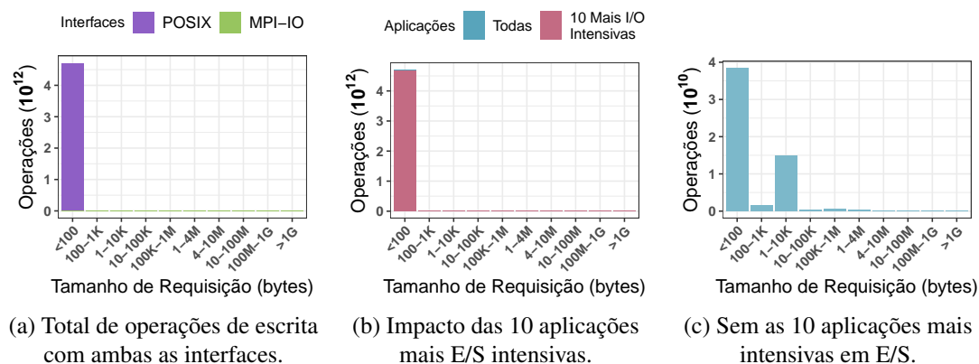
Figura 2. Análise das requisições de escrita. O eixo y possui diferentes escalas.
