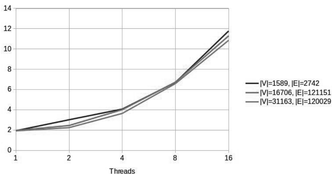
Figura 1. Speedup obtido para as instâncias de grafos da Tabela 1
