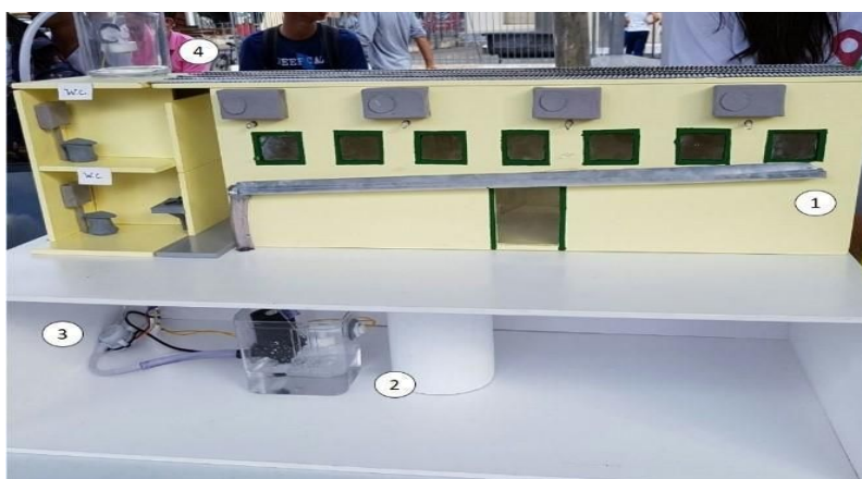
Figura 8. Resultado final da maquete.
