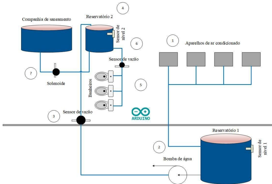
Figura 6. Planta de funcionamento da maquete.
