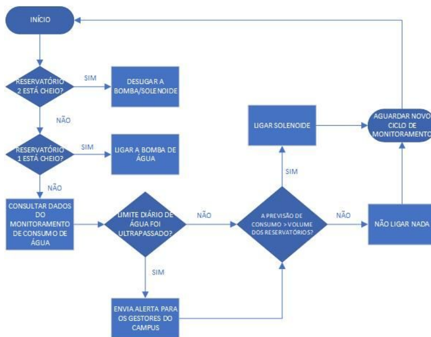
Figura 5. Fluxograma de funcionamento do sistema de monitoramento de consumo de água.
