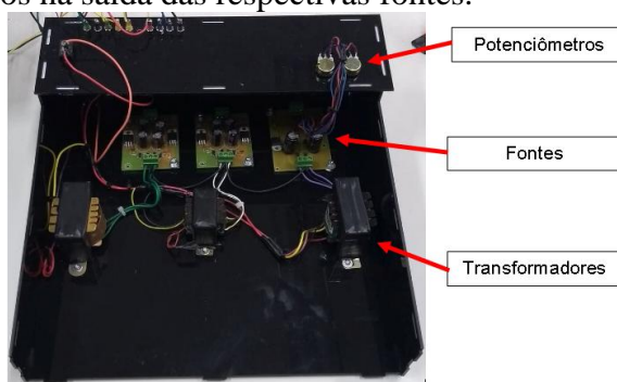
Figura 4. Fontes de tensão.
