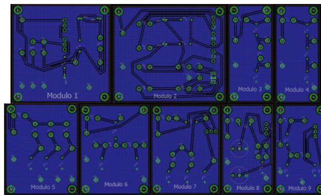
Figura 2. Layout da placa desenvolvido no software Eagle.
