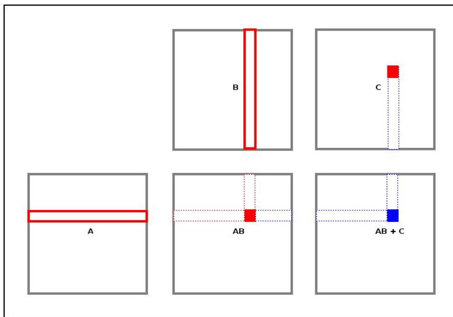
Figura 1. Representação simplificada da multiplicação de matrizes implementada pela rotina DGEMM
