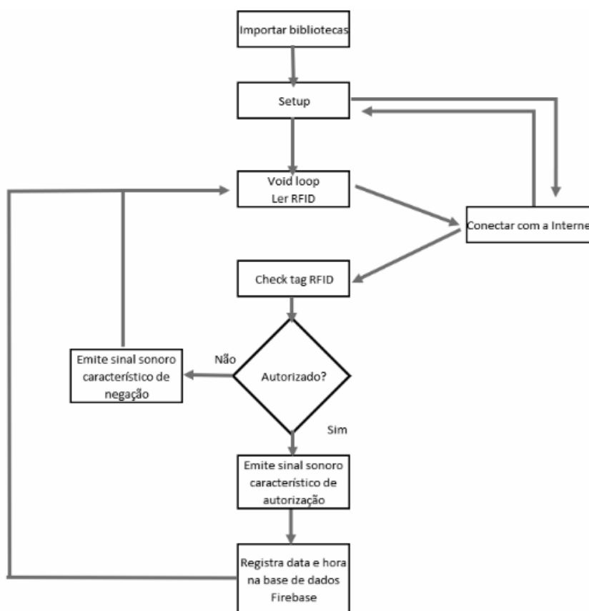
Figura 3 — Fluxograma do código no ESP32.
