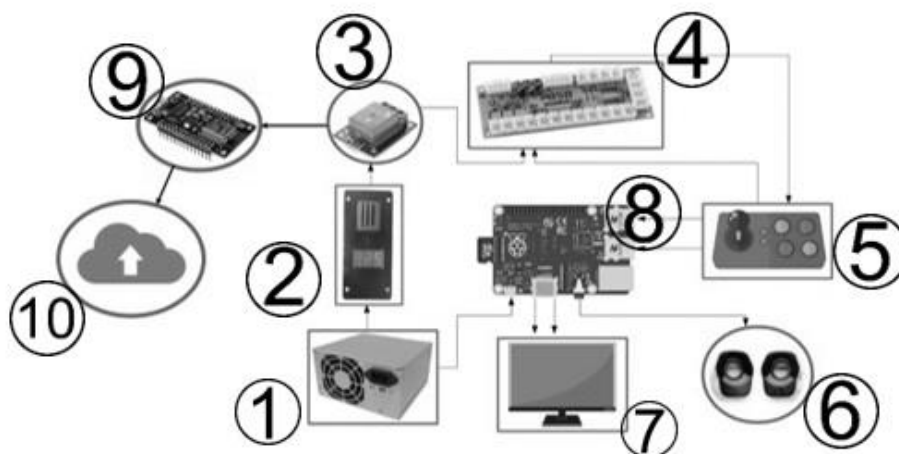
Figura 1. Esquemático geral do sistema desenvolvido.
