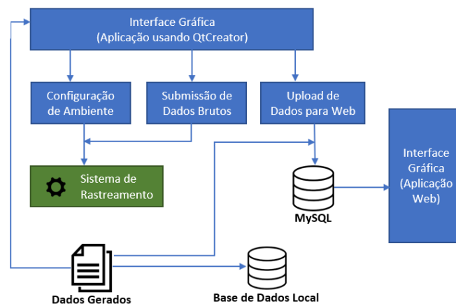
Figura 1. Arquitetura do FishTracker (Fonte: Autor)
