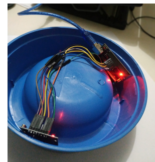
Figura 6. Protótipo do comedouro
