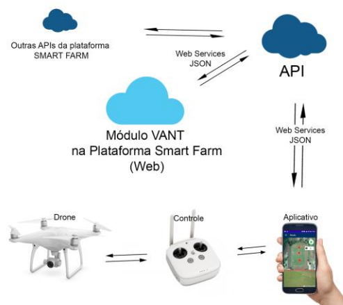
Figura 3. Arquitetura do módulo VANT
