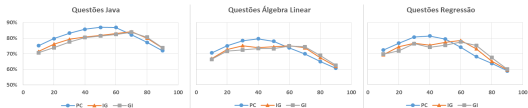
Figura 6. Acurácia X Filtro Naive Bayes
