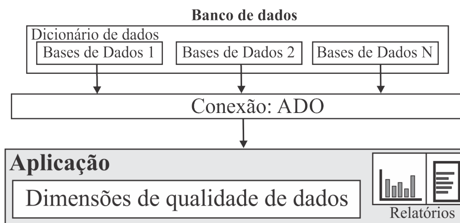
Figura 1. Arquitetura do protótipo.
