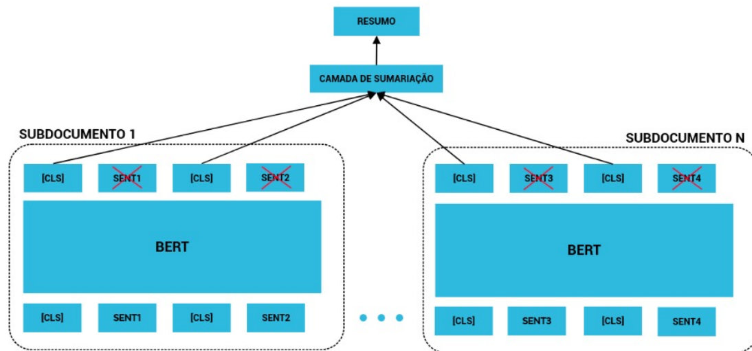
Figura 1. Modelo BertSum com entrada variada.
