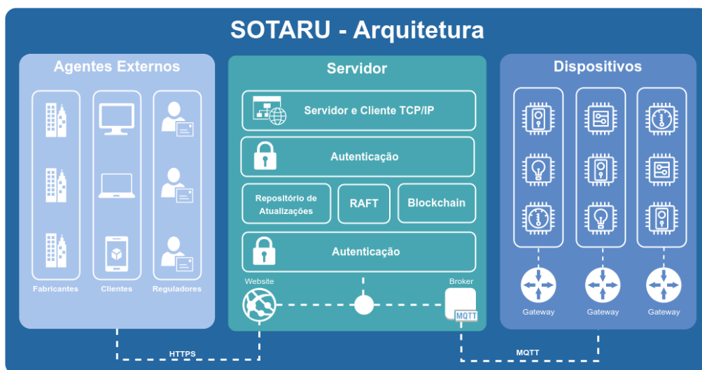
Figura 2. Arquitetura da Abordagem SOTARU
