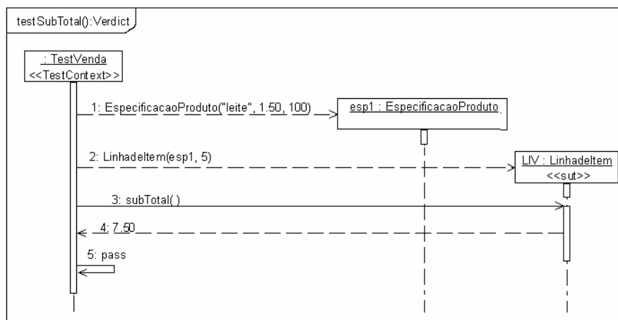
Figura 4. Comportamento do caso de teste testSubTotal .
