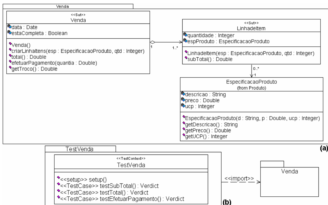
Figura 3. Projeto de Software e Projeto de Teste U2TP.
