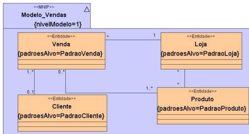
Figura 5. Modelo de Negócio Independente de Plataforma <<MNIP>> Modelo de Vendas
