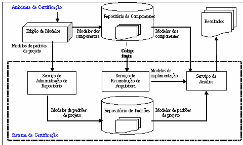
Figura 4. A Arquitetura conceitual do ambiente de certificação.
