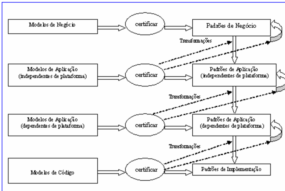
Figura 2. As certificações realizadas nos diversos níveis de abstração.
