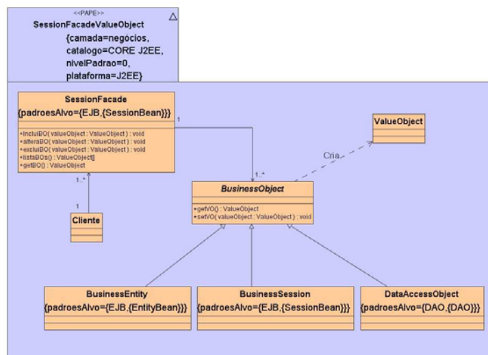
Figura 11. Padrão da Plataforma J2EE : SessionFacadeValueObject
