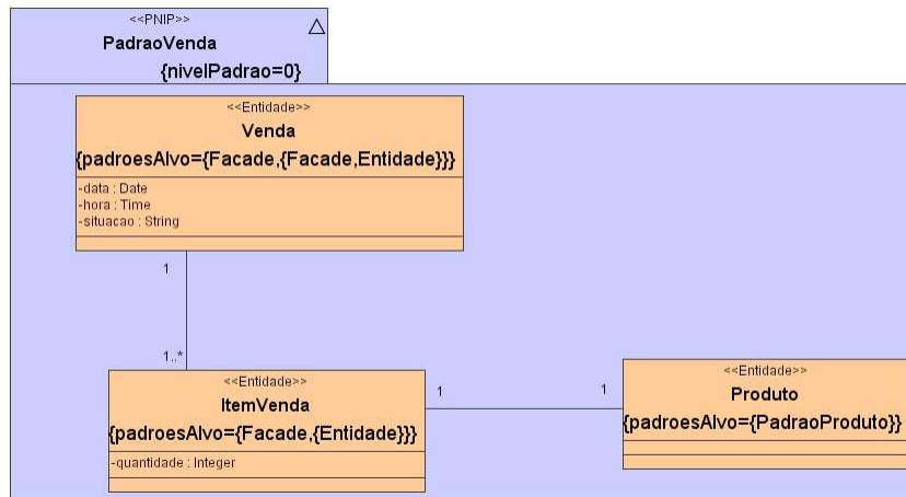
Figura 6. Padrão de Negócio Independente de Plataforma <<PNIP>> PadrãoVenda
