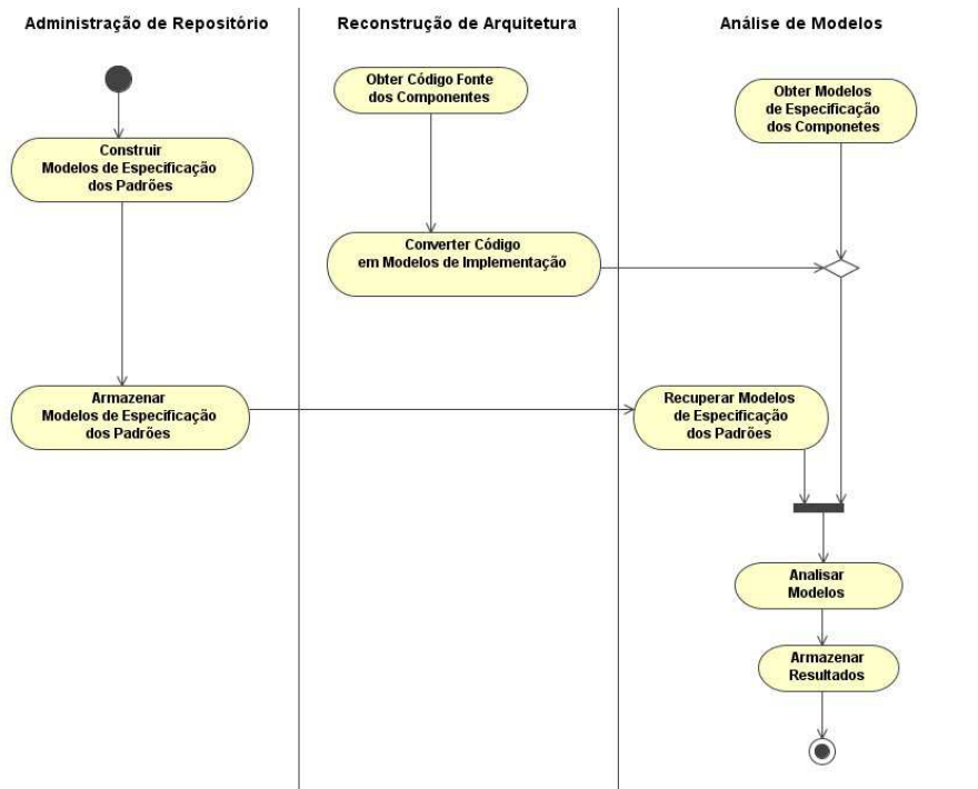
Figura 3. Diagrama de Atividades organizado por macro-atividades
