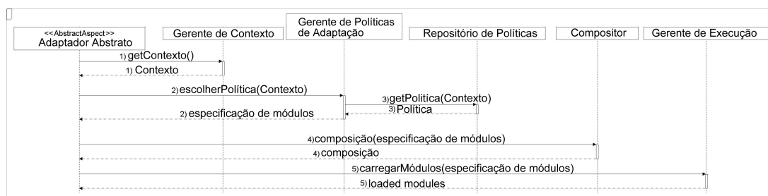
Figura 3. Diagrama de Seqüência parcial do PACCA
