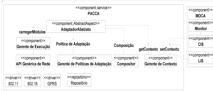
Figura 1 - Componentes do PACCA e sua integração com o MOCA
