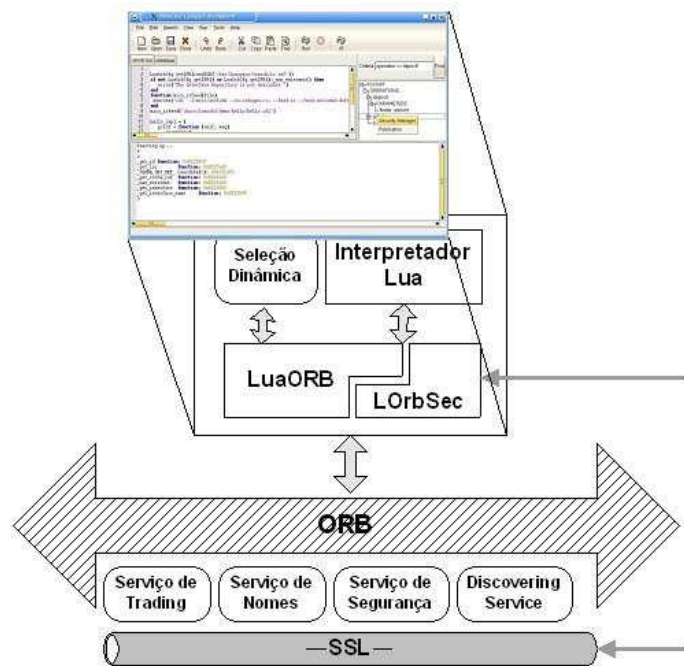
Figura 1 – Visão Geral de LuaSpace Plus
