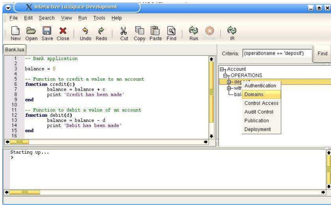
Figura 4 – Interface Gráfica do Ambiente LuaSpace Plus
