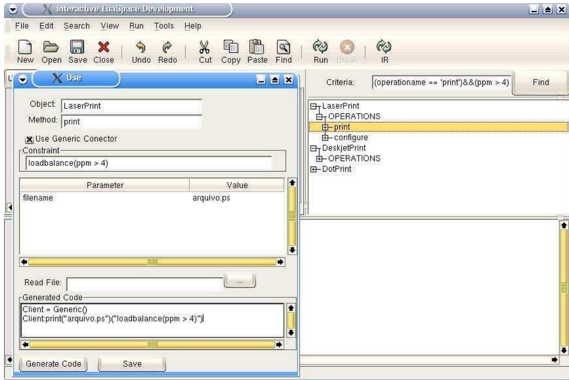
Figura 9 – Utilizando implementação do servidor de impressão
