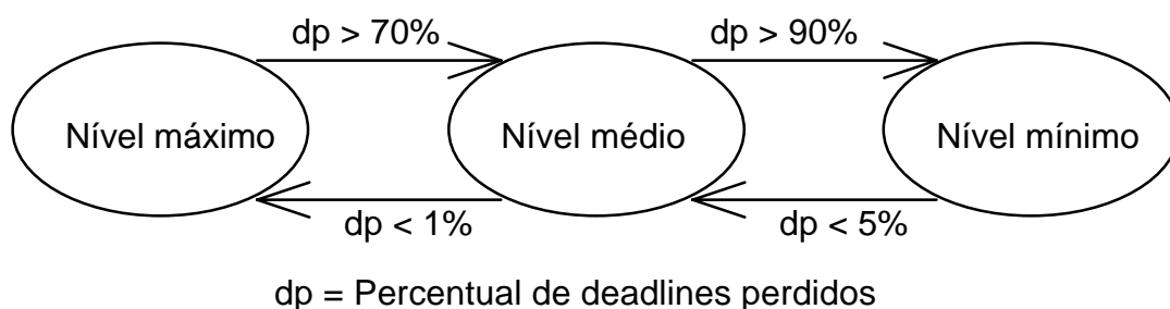
Figura 1 - MOE estruturado como uma máquina de estados.
