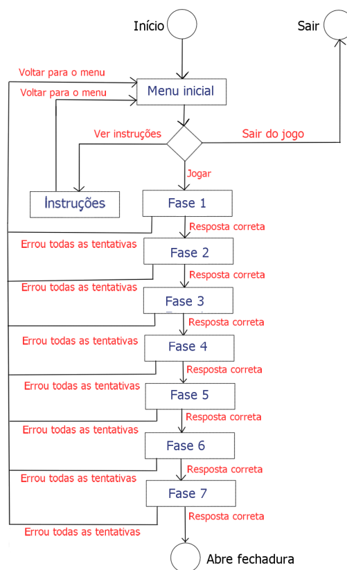
Fig. 1. Fluxograma da lógica do jogo.
