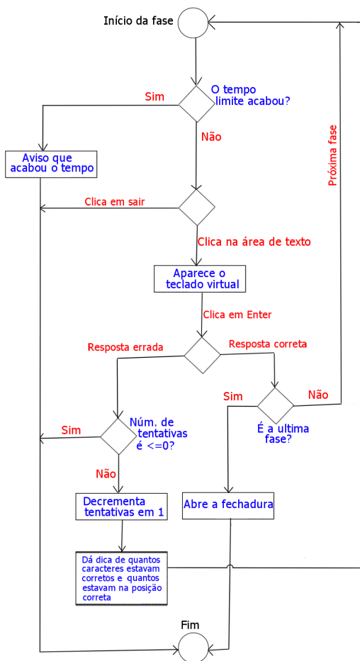
Fig. 2. Fluxograma da lógica de cada fase do jogo.
