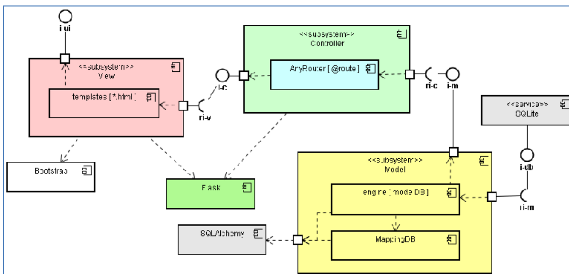
Figura 3 - Diagrama de componentes da versão construída
