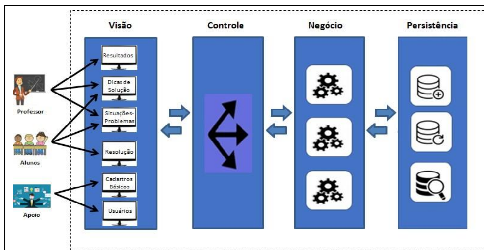
Figura 2: Arquitetura em camadas do ambiente proposto
