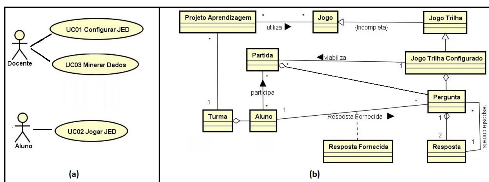
Figura 1. Modelos Parciais: (a) Funcional e (b) de Dados do “Jogo da Trilha”.
