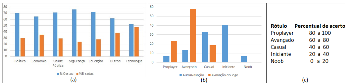
Figura 3. (a) Acerto/erro por tema (b) Autoavaliação e desempenho real (c) Faixas
