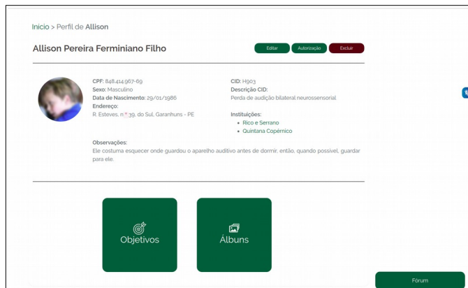
Figura 1. Interface para gerenciamento de aluno (dados fictícios)
