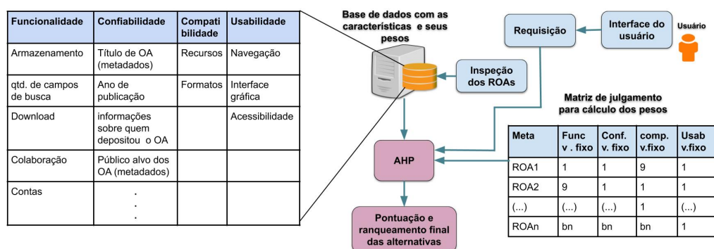
Figura 1. Arquitetura do Método de Avaliação de ROAs
