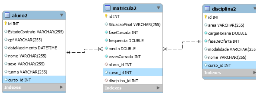
Figura 1. Diagrama Entidade Relacionamento
