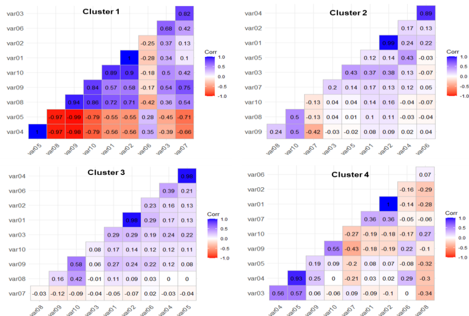
Figura 3. Matrizes de correlação para os Clusters do EF
