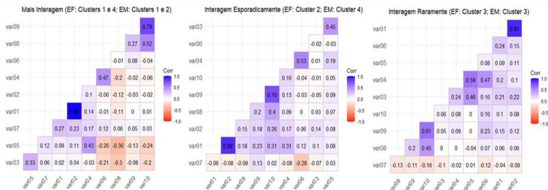
Figura 6. Correlação das variáveis para os níveis de interação
