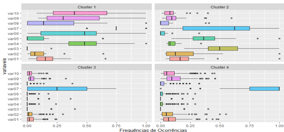
Figura 4. Frequência de ocorrência por variáveis para os Clusters do EM
