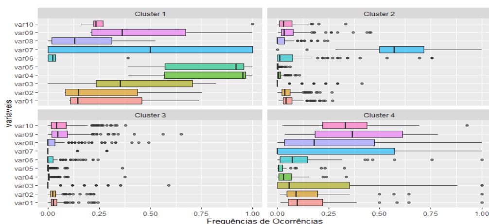
Figura 2. Frequência de ocorrência por variáveis para os Clusters EF
