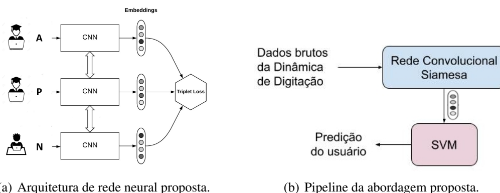
Figura 1. Método proposto. Os vetores de embeddings extraídos pela rede siamesa são utilizados pelo classificador SVM.
