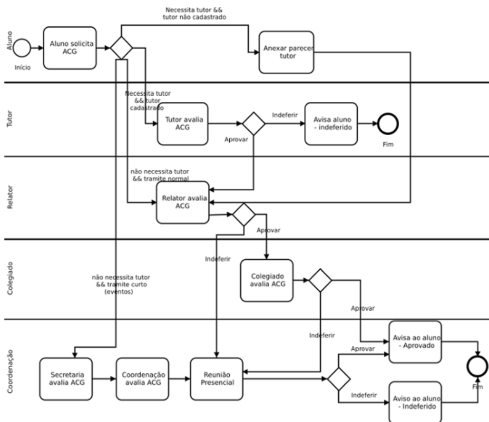
Figura 1. Diagrama do processo em BPMN
