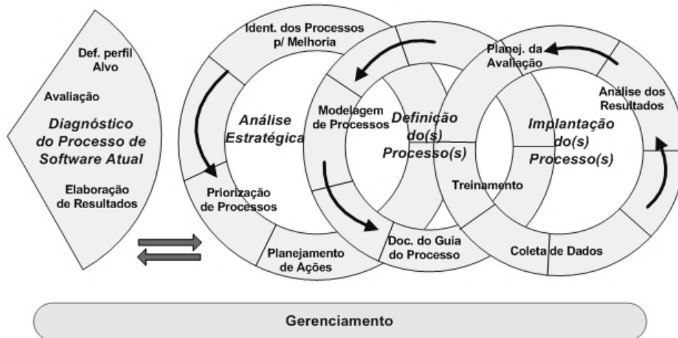
Figura 1: Visão geral da abordagem ASPE/MSQ
