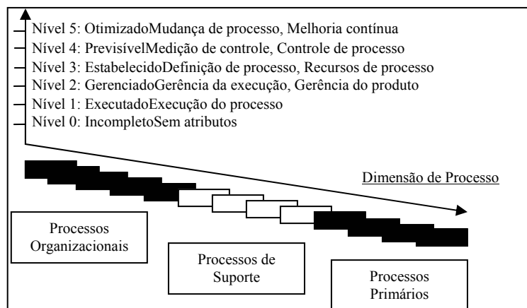
Figura 1: Dimensões da ISO/IEC 15504
