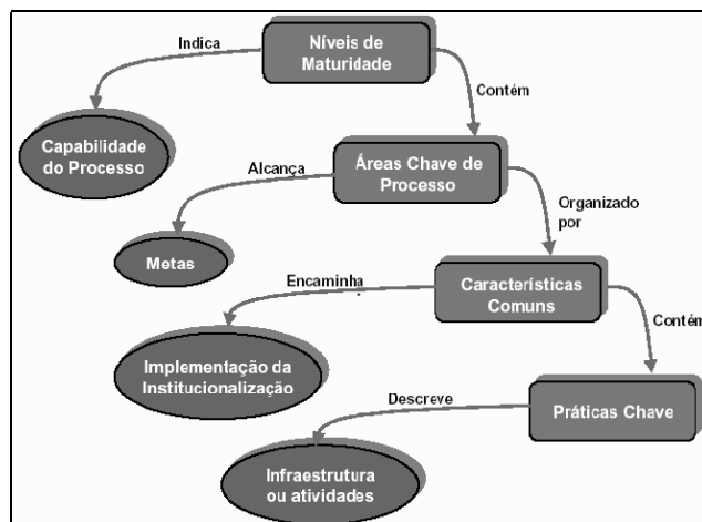
Figura 1 - Estrutura dos níveis de maturidade do SW-CMM
