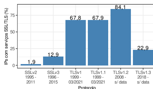
Figura 6. Versões de protocolos SSL/TLS.
