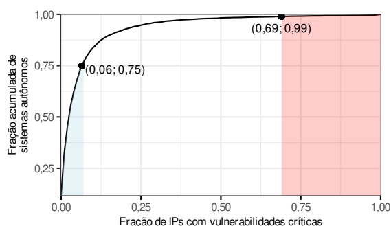
Figura 4. Prevalência de IPs com vulnerabilidades em um AS.
