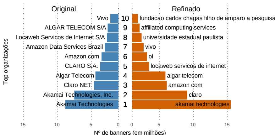
Figura 2. Diferença de resultado na identificação das top 10 organizações, em número de registros, entre o dataset original e padronização proposta.
