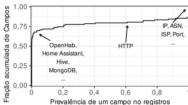
Figura 1. Prevalência dos campos nos registros do dataset.
