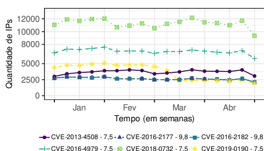
Figura 5. Vulnerabilidades em protocolos SSL/TLS.
