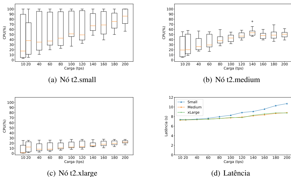
Figura 4. Uso de CPU e latência em nó da plataforma Ethereum.
