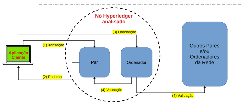
Figura 3. Componentes e fluxo de transações na plataforma Hyperledger Fabric.
