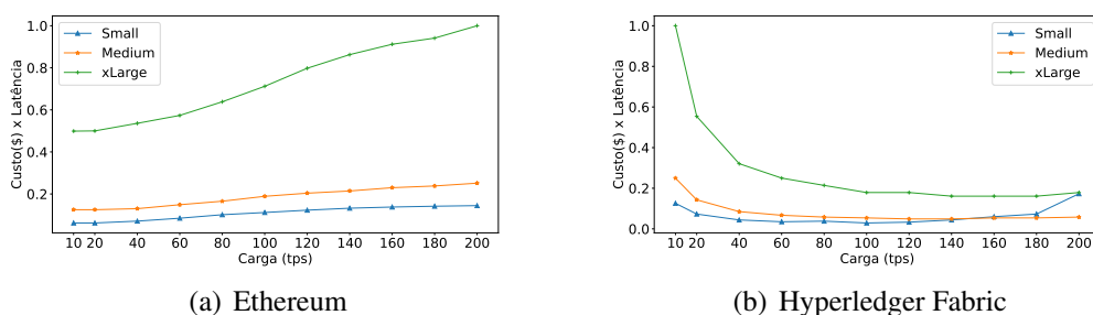
Figura 6. Compromisso entre custo e desempenho (normalizado) por nó em função da carga: melhores compromissos são os valores menores das curvas.
