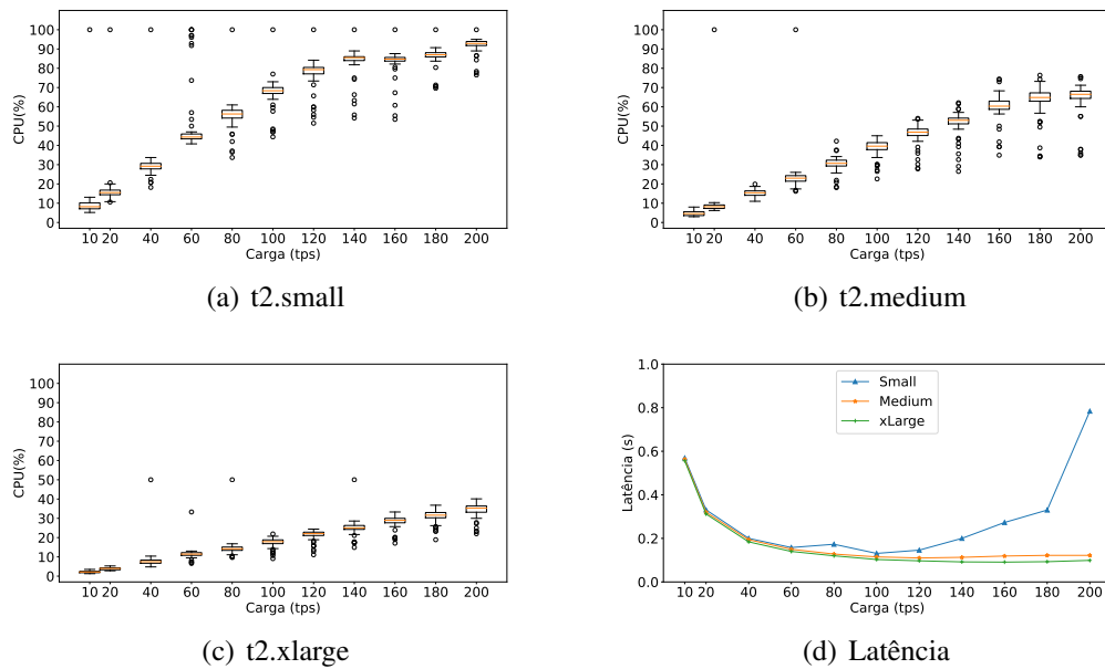
Figura 5. Uso de CPU e latência em rede permissionada Hyperledger Fabric.
