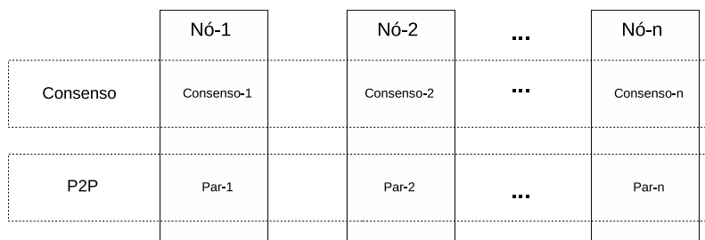
Figura 1. A arquitetura geral para um nó da rede blockchain pública ou permissionada.
