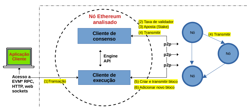
Figura 2. Modelo de rede pública Ethereum
